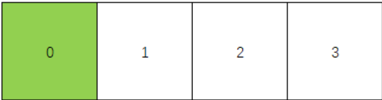
图 6-10 调度节点
