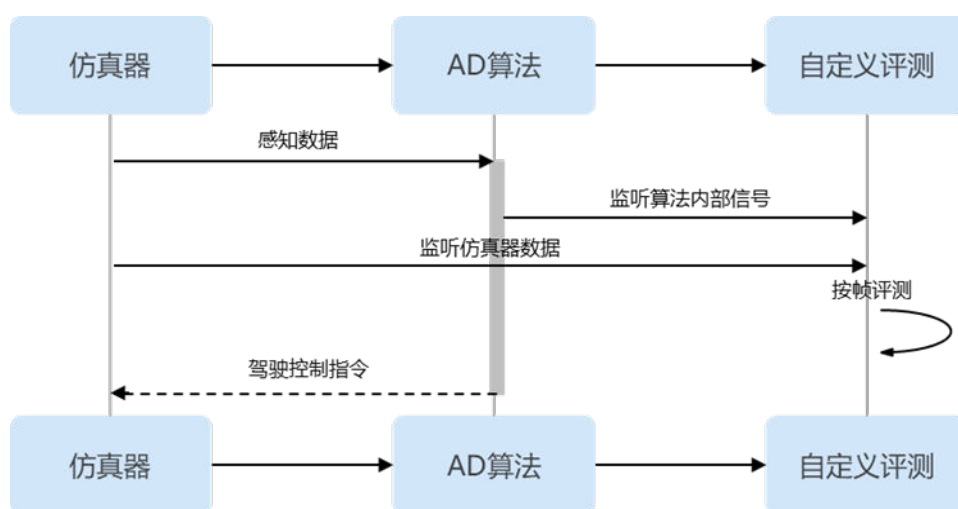
图 8-6 实时评测
