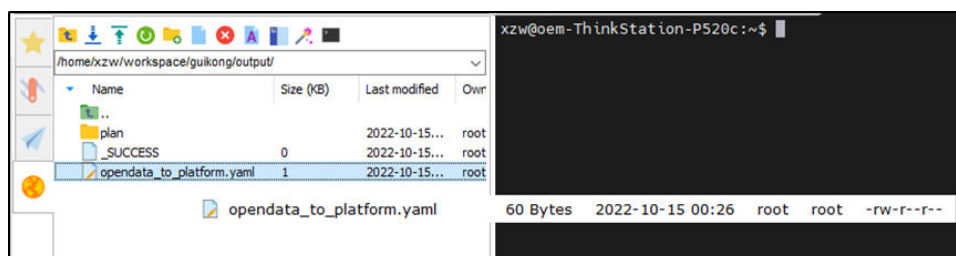
图 3-27 输出结果
