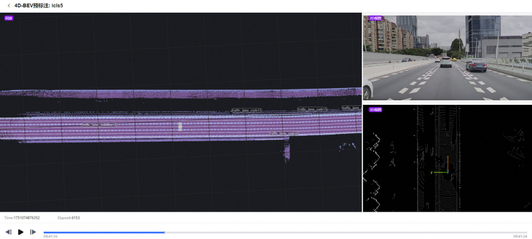
图 7-1 任务预览
