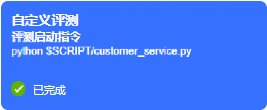
图 5-9 自定义评测
