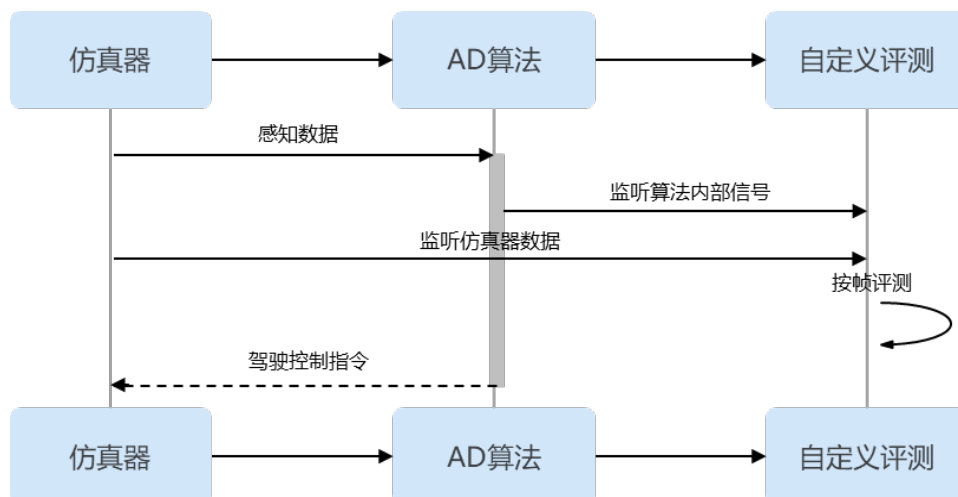
图 6-2 实时评测
