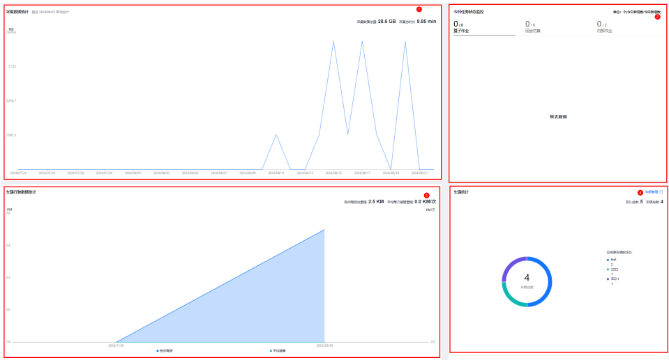
图 2-2 数据总览
