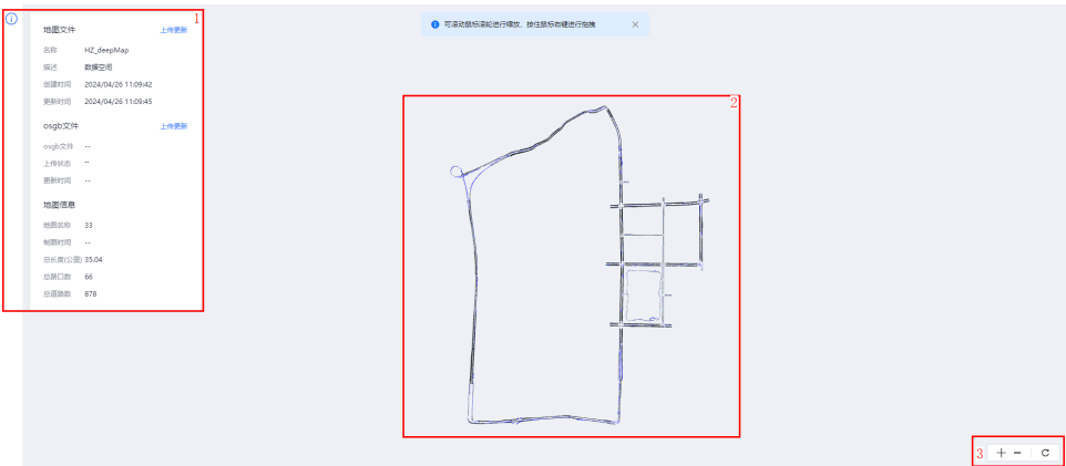
图 2-3 地图包详情
