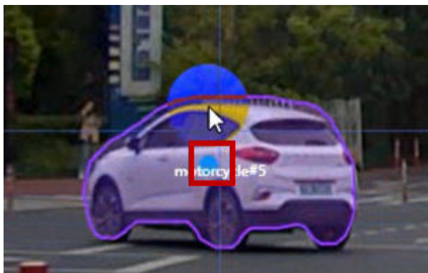
图 4-8 单击正点
