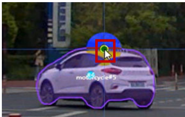
图 4-9 单击负点
