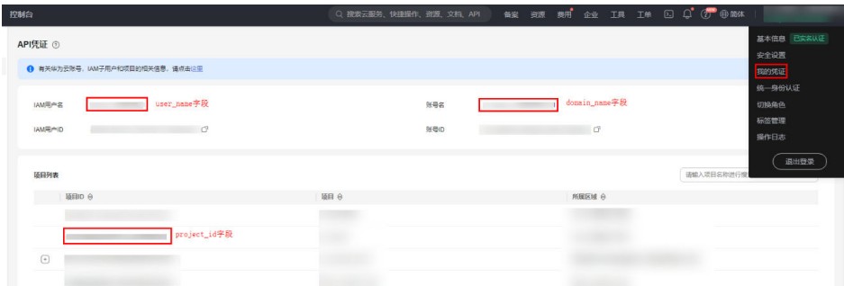
图 5-17 获取参数值
