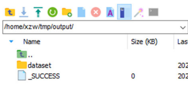
图 3-19 运行结果
