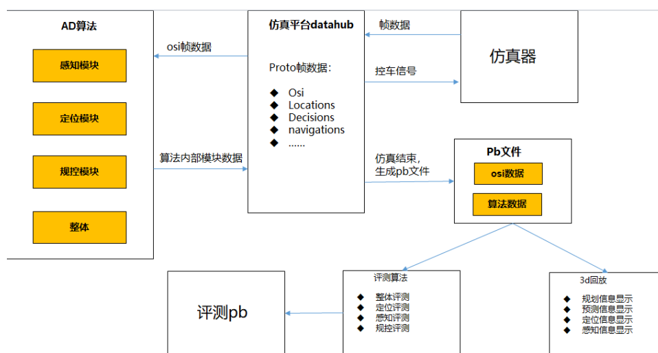
图 8-7 算法镜像
