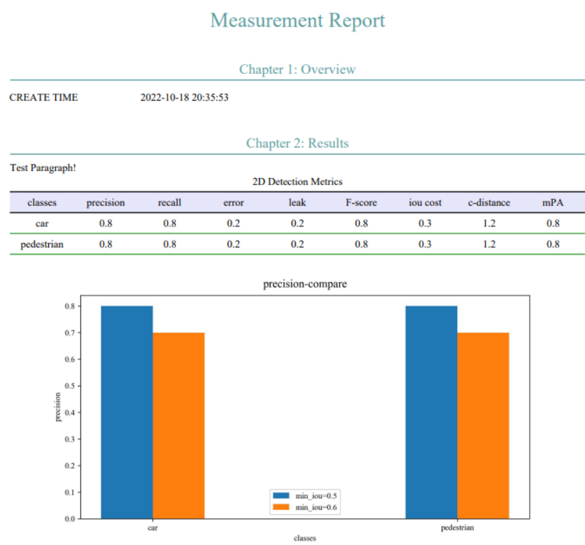
图 5-14 英文 pdf
