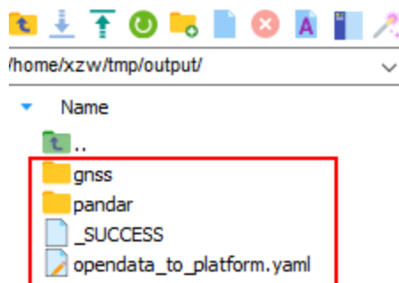
图 3-10 运行结果
